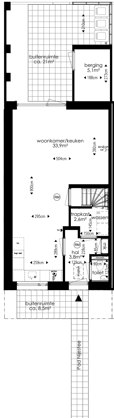
Begane grond
